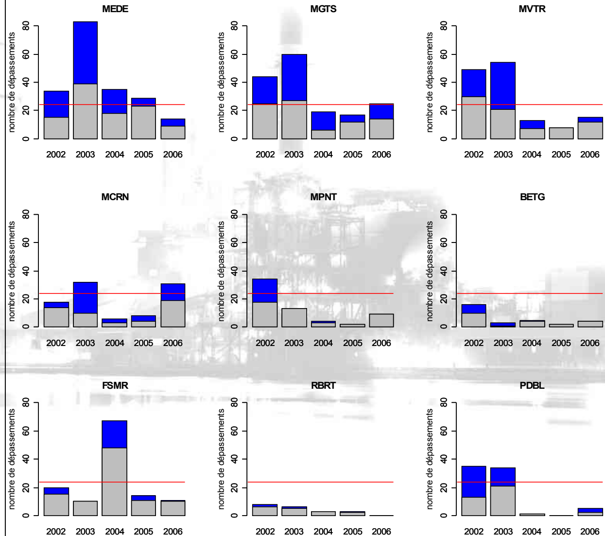
Répartition annuelle des dépassements du 350 \mu\text{g}/\text{m}^3 /heure observés et détectés
