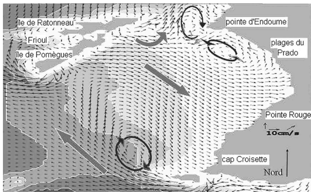
Fig. 7. Carte des courants de fond induits par un vent de SE 120^\circ - 10 \text{ m s}^{-1} .
