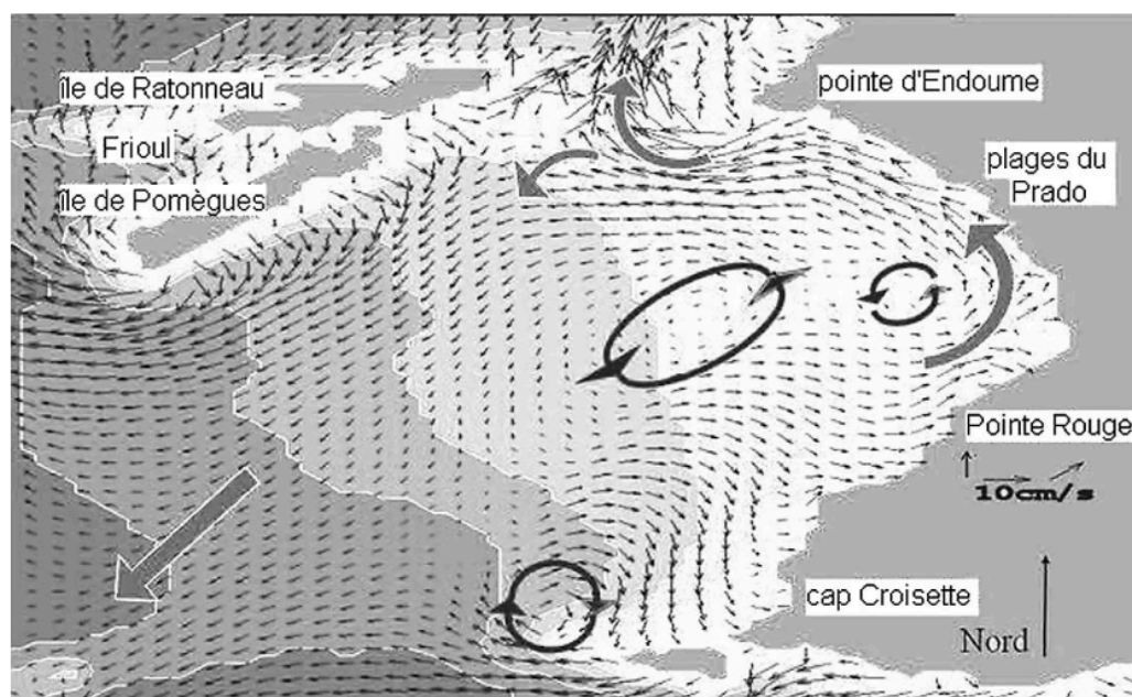
Fig. 8. Carte des courants de fond induits par un vent de SE 160^\circ - 10 \text{ m s}^{-1} .
