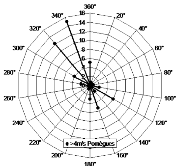
Fig. 2. Rose fréquentielle d'occurrence des vents de vitesse supérieure à 4 \text{ m s}^{-1} mesurés au sémaphore de Pomègues de 1976 à 1998.
