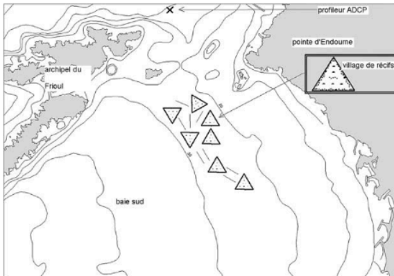
Fig. 1. Carte du domaine d'étude dans la baie sud de Marseille, avec la zone d'immersion des récifs artificiels constituée de sept « villages » juxtaposés.
