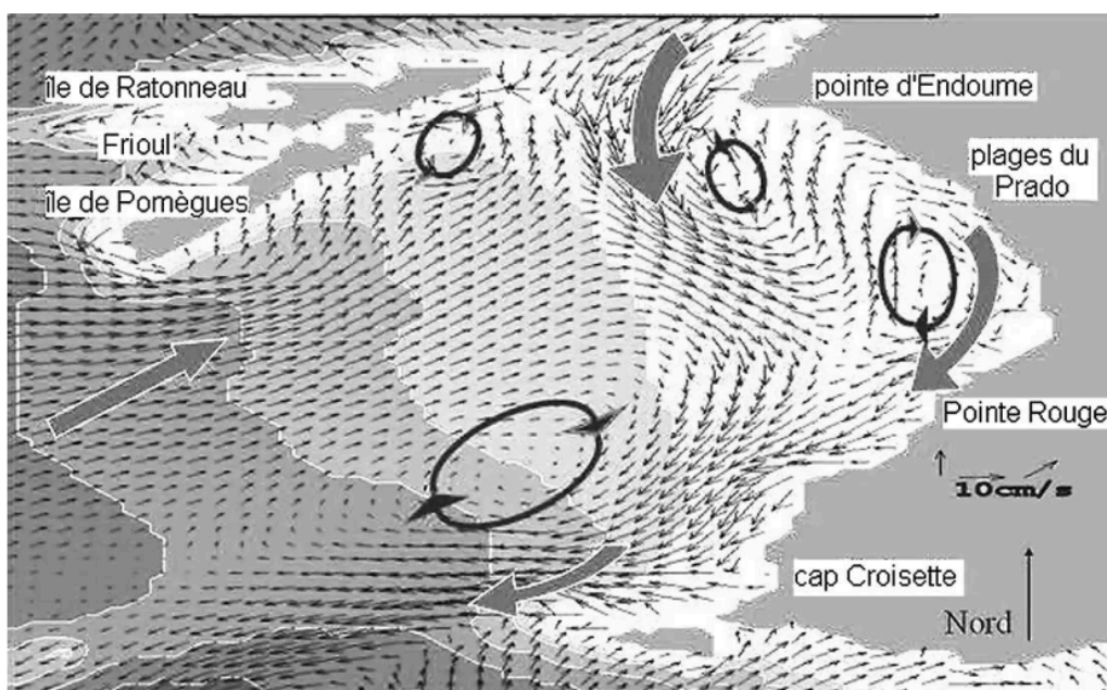
Fig. 6. Carte des courants de fond induits par un vent de NW 340° – 10 m s -1 .
