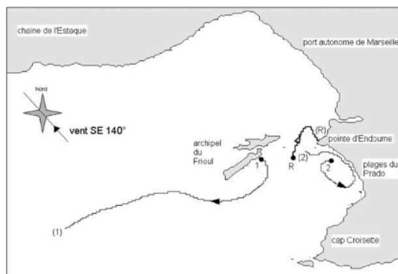
Fig. 11. Trajectoires des particules émises sur le fond sous un vent de SE 140^\circ - 10 \text{ m s}^{-1} . R et (R) : points de départ et d'arrivée des particules émises au niveau des récifs, 1 et (1) : points de départ et d'arrivée des particules émises à l'est du Frioul, 2 et (2) : points de départ et d'arrivée des particules émises au niveau de l'herbier de posidonies du Prado.
