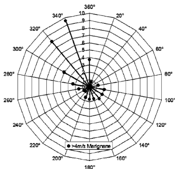
Fig. 3. Rose fréquentielle d'occurrence des vents de vitesse supérieure à 4 \text{ m s}^{-1} mesurés à l'aéroport de Marignane de 1971 à 2000.
