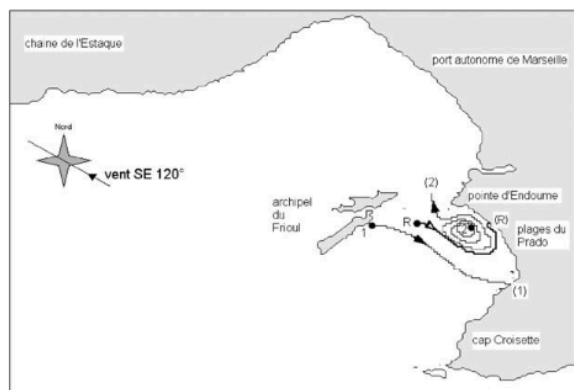
Fig. 9. Trajectoires des particules émises sur le fond sous un vent de SE 120^\circ - 10 \text{ m s}^{-1} . R et (R) : points de départ et d'arrivée des particules émises au niveau des récifs, 1 et (1) : points de départ et d'arrivée des particules émises à l'est du Frioul, 2 et (2) : points de départ et d'arrivée des particules émises au niveau de l'herbier de posidonies du Prado.
