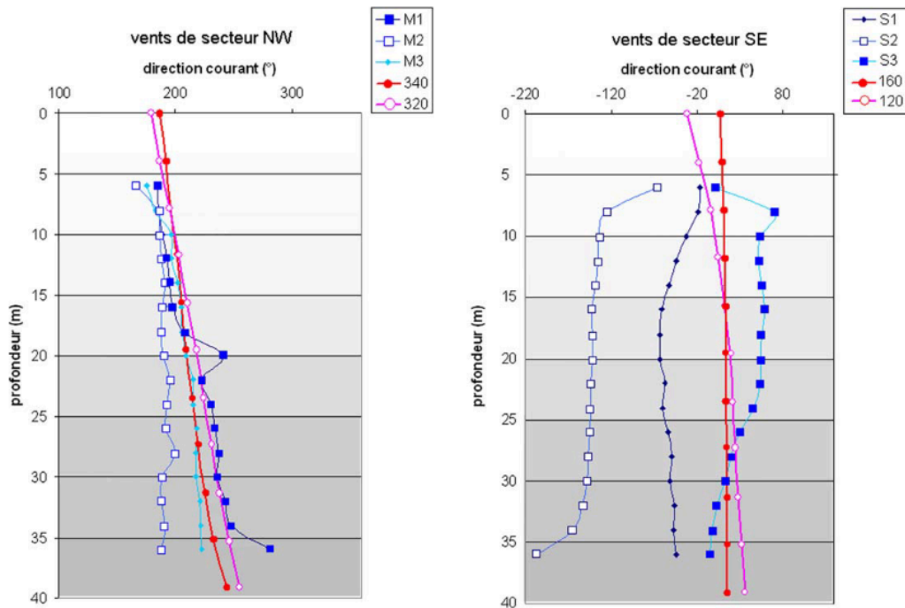
Fig. 4. Validation en direction des profils des courants simulés par vents de NW (320°, 340°) et SE (120°, 160°) par comparaison avec les courants mesurés par vents de NW (M1, M2, M3) et SE (S1, S2, S3) respectivement.
