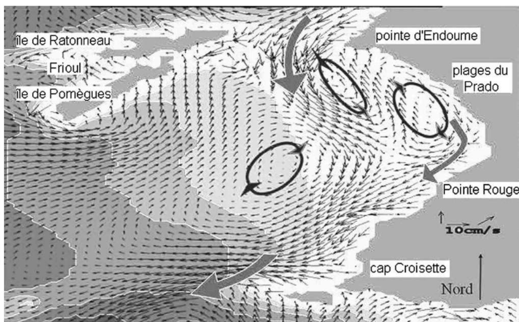
Fig. 5. Carte des courants de fond induits par un vent de NW 320° – 10 m s -1 .
