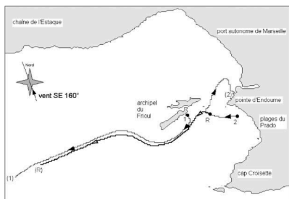
Fig. 10. Trajectoires des particules émises sur le fond sous un vent de SE 160^\circ - 10 \text{ m s}^{-1} . R et (R) : points de départ et d'arrivée des particules émises au niveau des récifs, 1 et (1) : points de départ et d'arrivée des particules émises à l'est du Frioul, 2 et (2) : points de départ et d'arrivée des particules émises au niveau de l'herbier de posidonies du Prado.
